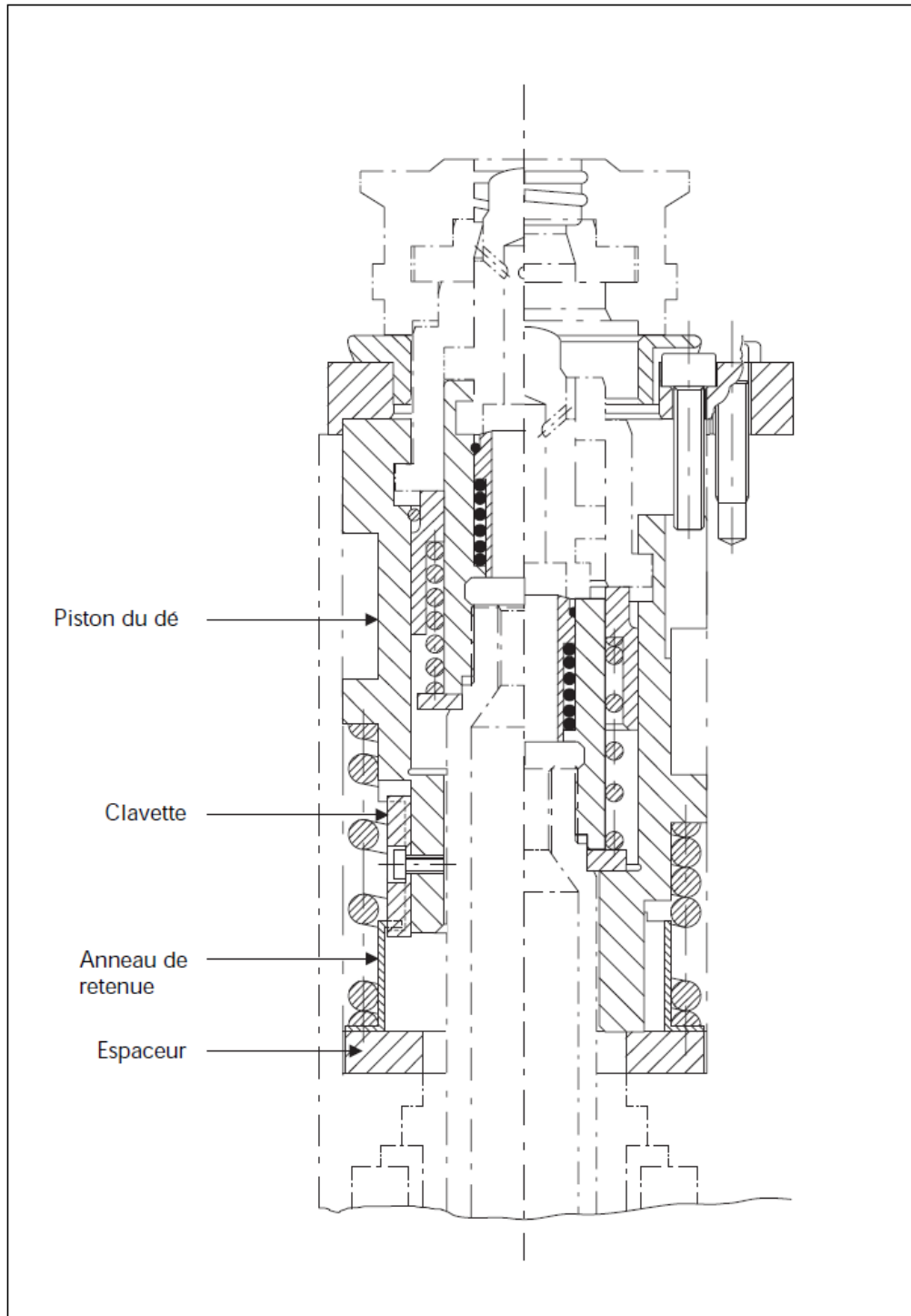
Fig. 1: Cartouche à changement rapide 62-3051 Groupe 10 montre
