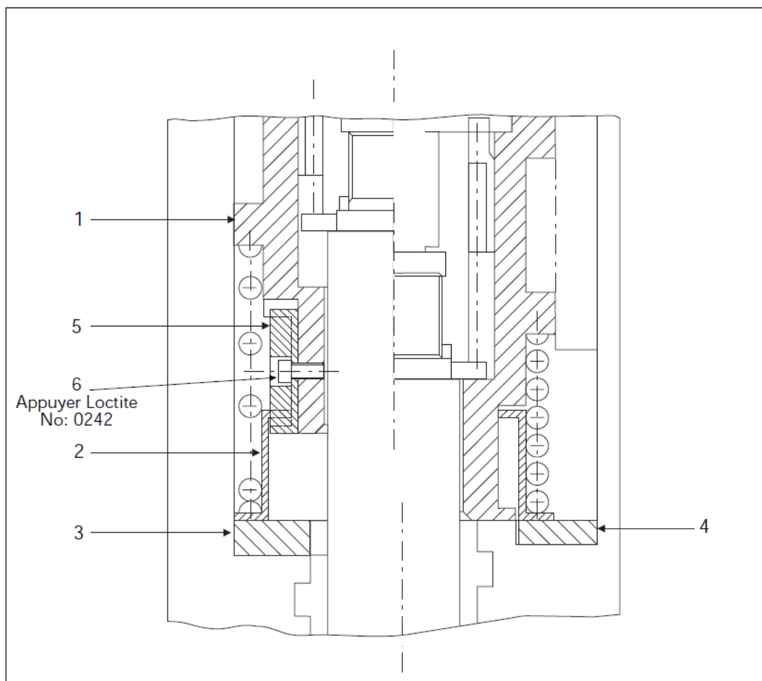
Fig. 2: Conversion de la Cartouche 62-D 3051
